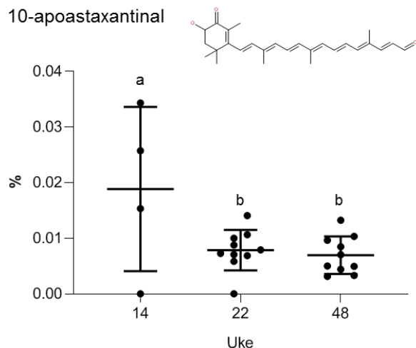
Figur 8. Astaxantin oksidasjonsprodukter relativ til total astaxantin i laksemuskel (%). Forholdet ble bestemt med LC-TWIMS-QTOF, og prøver fra uke 14 (april), uke 22 (juni) og uke 48 (desember) ble analysert. 10-apoastaxantinal i uke 14 var signifikant høyere ( p < 0.05 ) enn i uke 22 og 48. 14-apoastaxantinal i uke 14 og 22 var signifikant høyere enn i uke 48 ( p < 0.05 ). Statistisk analyse utført i GraphPad Prism, One-way ANOVA med Tukey's multiple comparison test.
