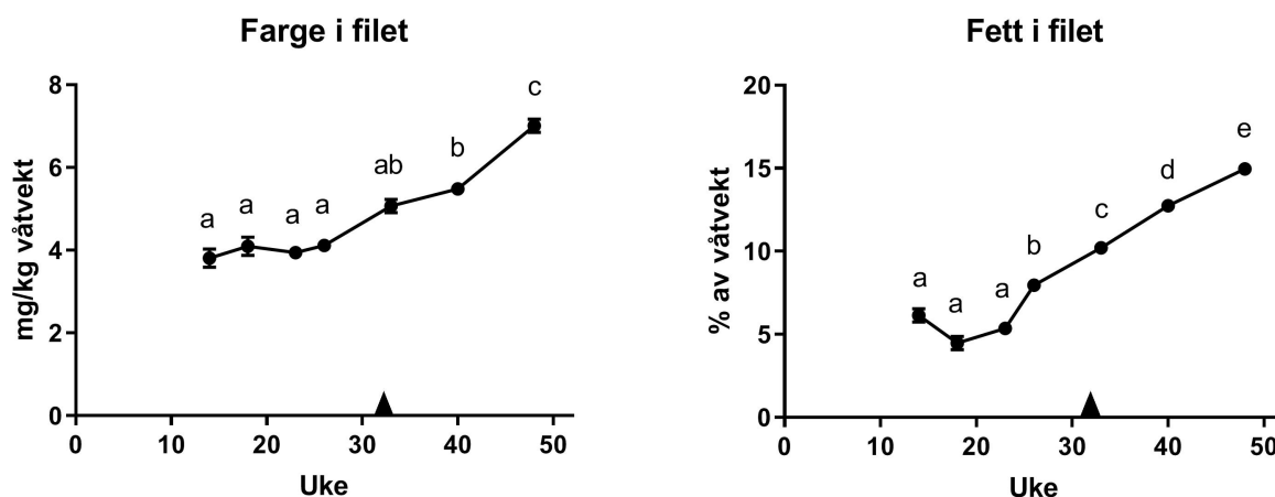
Figur 5. Farge og fett i filet per ukenummer i 2017 målt med Photofish (snitt±pooled SEM, n=12-20). Trekanten på x-aksen indikerer maksimum for temperatur og SGR. Signifikante forskjeller ( p<0.05 ) vises med ulike bokstaver.
