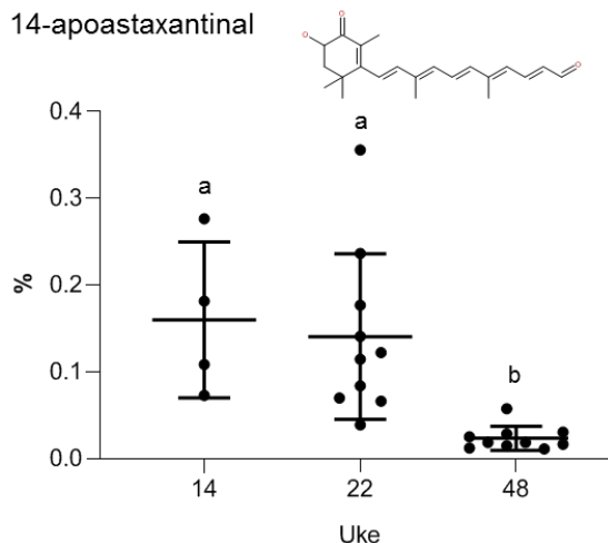
Figur 8. Astaxantin oksidasjonsprodukter relativ til total astaxantin i laksemuskel (%). Forholdet ble bestemt med LC-TWIMS-QTOF, og prøver fra uke 14 (april), uke 22 (juni) og uke 48 (desember) ble analysert. 10-apoastaxantinal i uke 14 var signifikant høyere ( p < 0.05 ) enn i uke 22 og 48. 14-apoastaxantinal i uke 14 og 22 var signifikant høyere enn i uke 48 ( p < 0.05 ). Statistisk analyse utført i GraphPad Prism, One-way ANOVA med Tukey's multiple comparison test.
