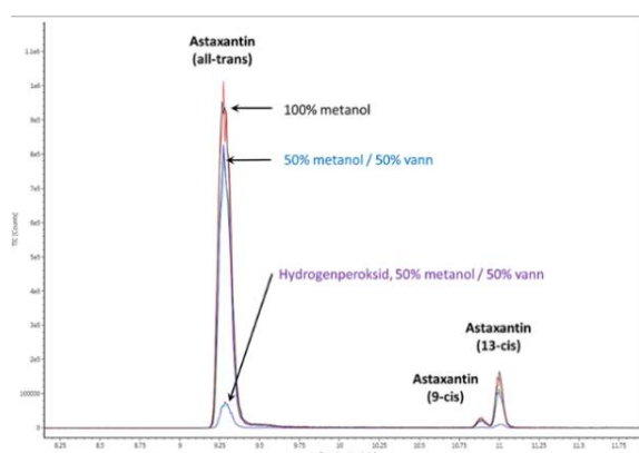
Figur 7.. LC-TWIMS-QTOF analyse av astaxantin standard og ekstraherte ionekromatogrammer. Ionokromatogrammene t.v. viser de tre kjente stereoisomerene av astaxantin, og mengden detektert når løst i metanol (kontroll), når løst i metanol tilsatt vann (kontroll) og når løst i metanol tilsatt vann og hydrogenperoksid (oksidert). Ionokromatogrammet t.h. viser at 14-apoastaxantinal kun ble detektert i prøven tilsatt hydrogenperoksid.
