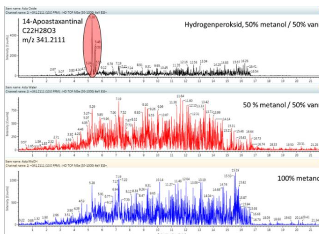
Figur 7.. LC-TWIMS-QTOF analyse av astaxantin standard og ekstraherte ionekromatogrammer. Ionokromatogrammene t.v. viser de tre kjente stereoisomerene av astaxantin, og mengden detektert når løst i metanol (kontroll), når løst i metanol tilsatt vann (kontroll) og når løst i metanol tilsatt vann og hydrogenperoksid (oksidert). Ionokromatogrammet t.h. viser at 14-apoastaxantinal kun ble detektert i prøven tilsatt hydrogenperoksid.
