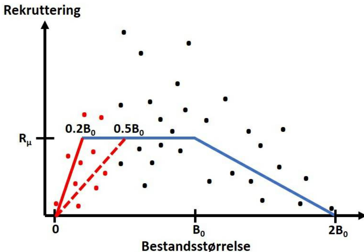
Figur 3. Illustrasjon av forholdet mellom rekruttering og bestandsstørrelse. Rekrutteringen blir redusert når størrelsen på bestanden minker eller går under en terskelverdi (50 % stipledd rød linje, og 20 % rød heltrukken linje). Rekrutteringen hvert år er en tilfeldig verdi utfra en fordeling som baseres på empiriske estimater av en gjennomsnittrekruttering R_\mu og en variasjon eksemplifisert her som svarte og røde punkter (tilsvarende til rekruttering over og under terskelverdien).
