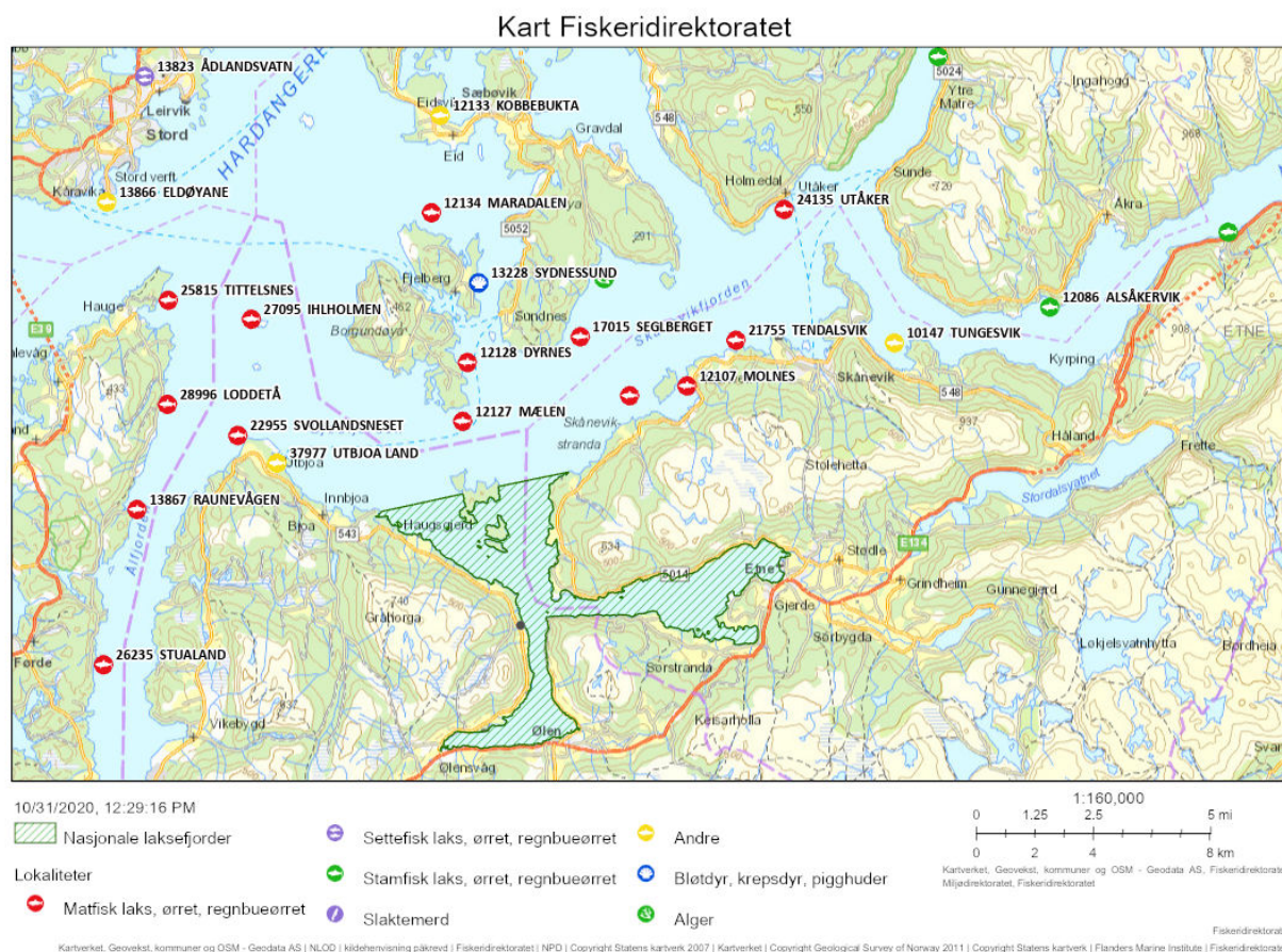
Figur 4.75: Kart som viser funnsted av død krill ved Vågå i Ølen i Ølsfjorden (markert med svart runding) 17. august 2018, med nærliggende oppdrettslokaliteter ( https://open-data-fiskeridirektoratet-fiskeridir.hub.arcgis.com/ ).
