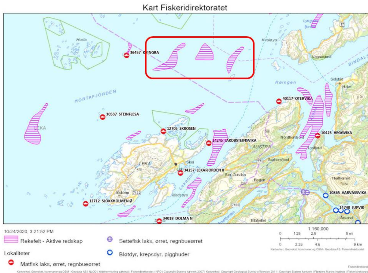
Figur 6.1. Rekefelt (innringet) der en rekefisker rapporterte at rekene forsvant etter tømning av avlusingsvann fra brønnbåt i november 2012 ( https://open-data-fiskeridirektoratet-fiskeridir.hub.arcgis.com/ ). Rekeprøven som ble sendt til Havforskningsinstituttet, ble tatt fra det midterste feltet (Midterfeltet) ( 65^{\circ} 12,15' N , 11^{\circ} 46,77' O ).
