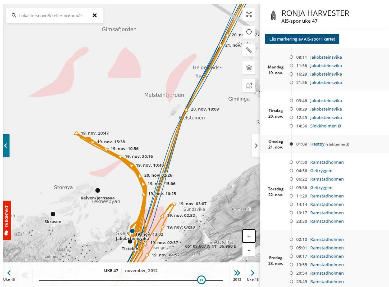
Figur 6.6: Brønnbåtaktivitet i Hortaafjorden i uke 47 i 2012 ( https://www.barentswatch.no/fiskehelse ). Brune streker viser AIS-spor fra Ronja Harvester.
