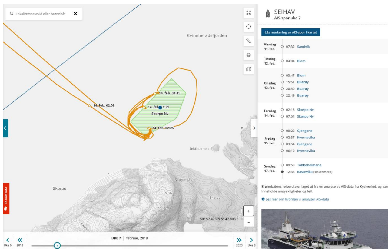
Figur 4.106: Brønnbåttaktivitet ved Skorpo Nv i uke 7 i 2019 ( https://www.barentswatch.no/fiskehelse/ ). Brune streker viser AIS-spor fra Seihav.
