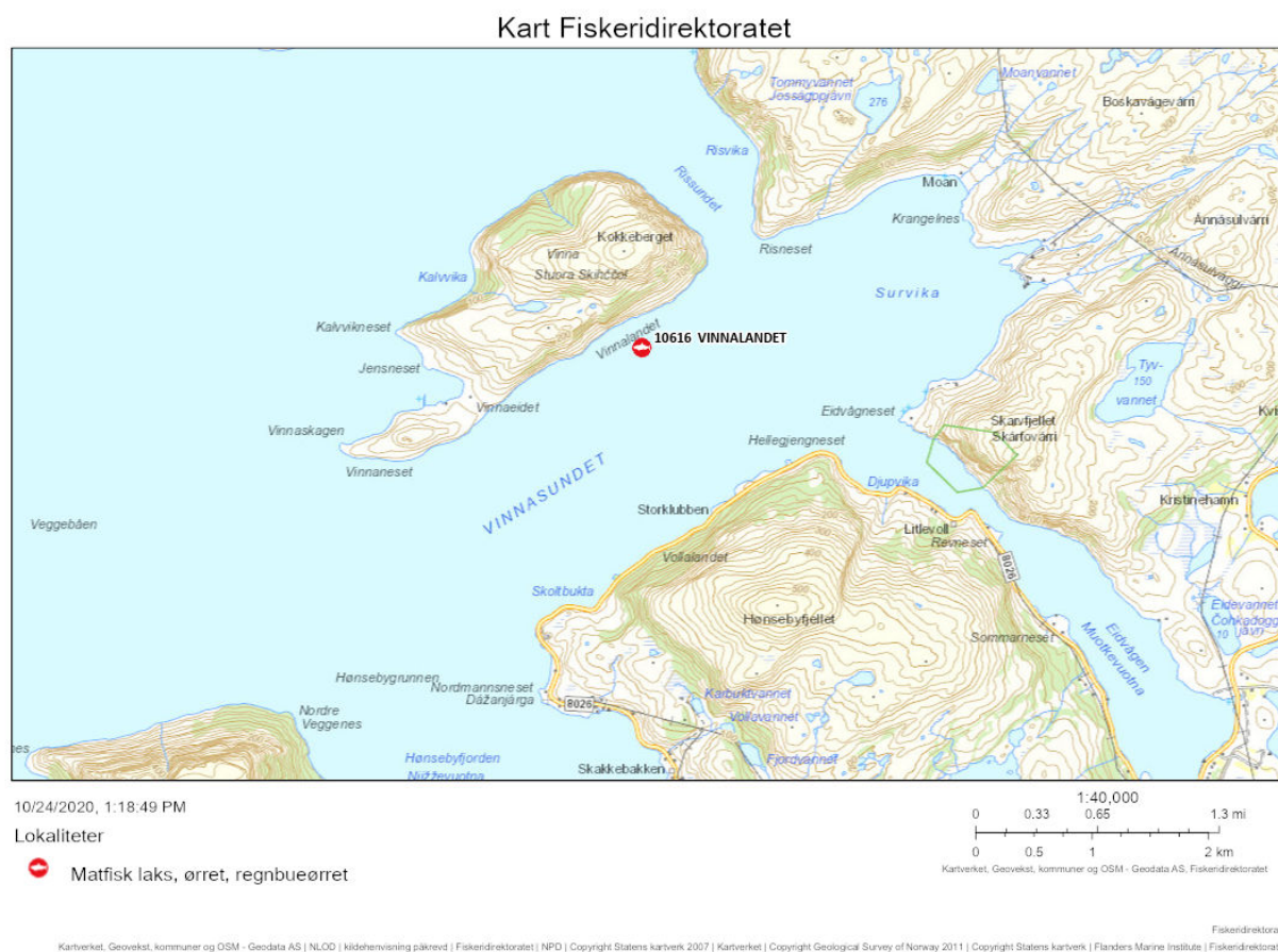
Figur 5.5: Kart over området hvor død raudåte ble observert våren 2017 ( https://open-data-fiskeridirektoratet-fiskeridir.hub.arcgis.com/ ).
