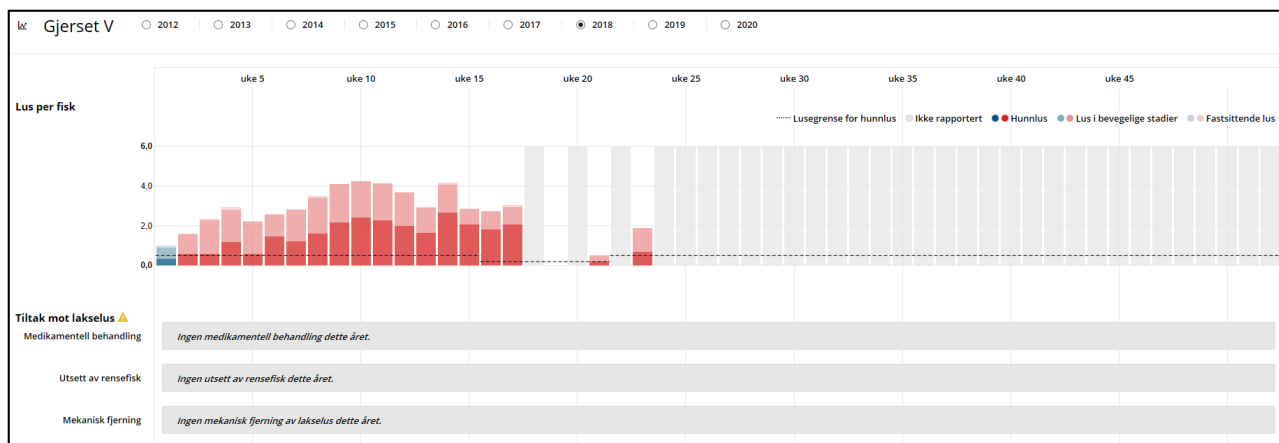
Figur 4.61: Lus per fisk og eventuell avlusingsmetode per uke i 2018 for stamfiskanlegget Gjerset V ( https://www.barentswatch.no/fiskehelse/ ). Funnet av død krill ble gjort i uke 11.
