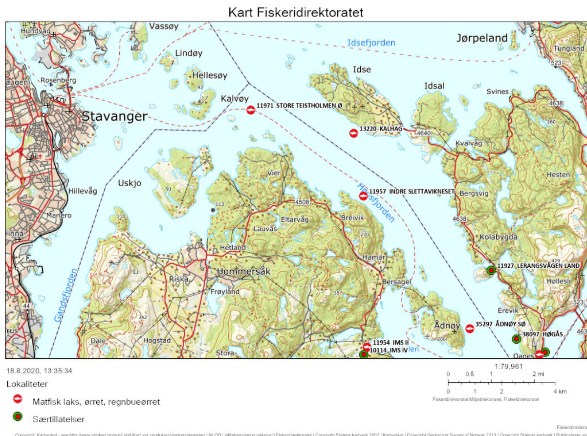
Figur 4.145: Kart som viser funnsted av død krill i Skjølvgå i Uskasundet i Sandnes kommune (markert med svart runding) i august 2020, med nærliggende oppdrettslokalteter ( https://open-data-fiskeridirektoratet-fiskeridir.hub.arcgis.com/ ).
