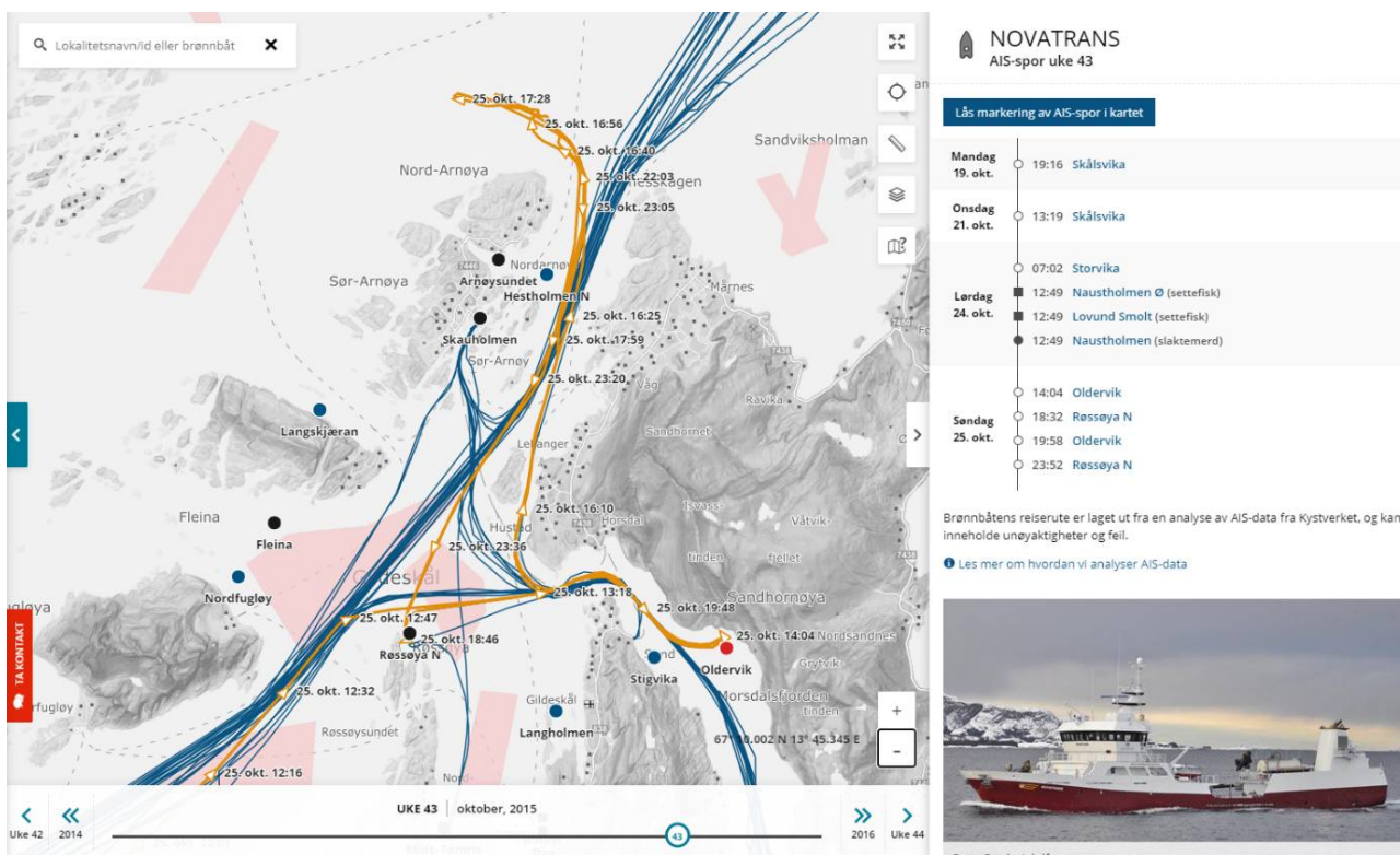
Figur 6.14: Brønnbåtkaktivitet i Gildeskål i uke 43 i 2015 ( https://www.barentswatch.no/fiskehelse ). Brune streker viser AIS-spor fra Novatrans.
