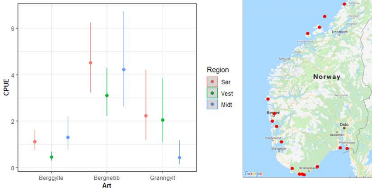
Figur 20. Venstre; Fangst per enhet innsats (CPUE) med 95 % konfidensintervall for de tre artene i de tre regionene i 2019, estimert ved GLMM. Høyre: Fordelingen av de 16 referanseciskerne i 2019.
