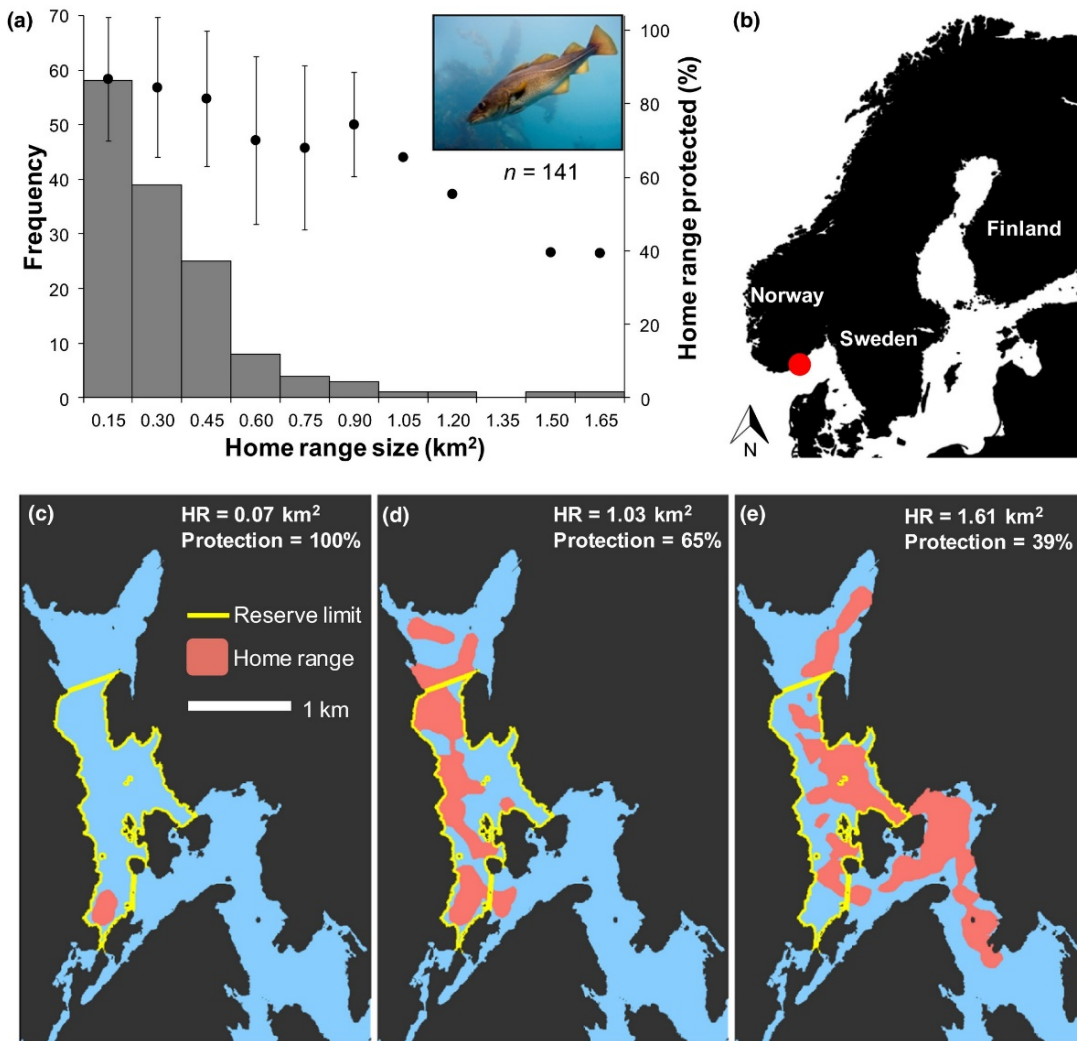
Figur 18. Hjemmeområde for torsk i Tvedestrandsfjorden. De fleste torsk har hjemmeområder på under en halv \text{km}^2 (a). I c, d og e vises eksempler på enkeltindividers hjemmeområder, der torsken i c har et mye mindre hjemmeområde enn d og e. Området er så lite at den er beskyttet til enhver tid av null-fiskeområdet. Kilde: Villegas-Rios mfl. 2016.
