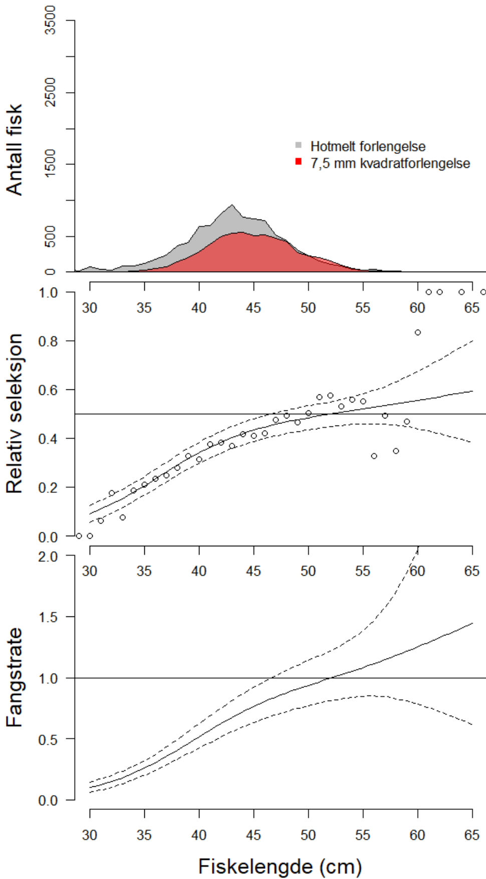
Figur 9. Størrelsesfordelinger for hyse i hver forsøksserie (topp) med 7 parvise hal. Relativ fangst i snurrevadsekk med 7,5 mm tråd i kvadratmaskeforlengelse, sammenlignet med sekk med diamantmaskeforlengelse (midt). Figuren nederst viser relativ fangstrate (fangsttap av fisk < ca 50 cm) ved å bruke kvadratmaskeforlengelse.
