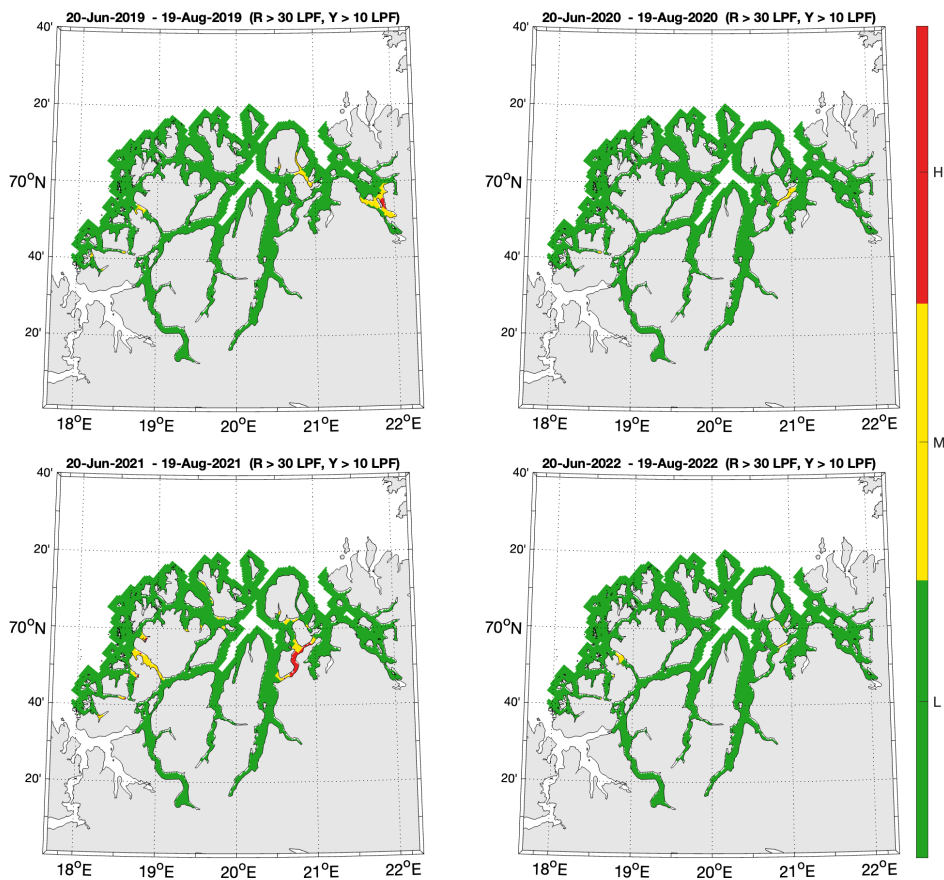
Figur 6.132. Kart som viser hvor det er forventet at postsmolt av ørret som beiter i området fra dato for median for smoltutvandring i produksjonsområdet (periode gitt i kartene) vil bli infisert med mer enn 18 mobile lus (rød), mellom 6-18 mobile lus (gul) og mindre enn 6 mobile lus (grønn).
