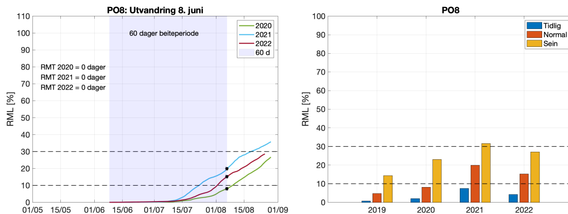
Figur 6.101. Venstre figur viser kumulativt redusert marint leveområde (RML) for fisk som utvandrer ved median dato for utvandring for alle elvene i produksjonsområdet og redusert marin beiteperiode (RMT) 2020-2022 (tekst i figuren). Skravert område indikerer antatt naturlig beiteperiode (60 dager). Høyre figur viser RML etter 60 dager for årene 2019-2022 ved median dato for utvandring (Normal), og ved 20 dager tidligere (Tidlig) eller 20 dager senere utvandring (Sein).
