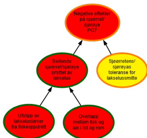
Figur 4.20. Visualisering av risikobilde for negative effekter på sjørøret som følge av utslipp av lakselus fra lakseoppdrett i produksjonsområde 7 (PO 7) Nord-Trøndelag.
