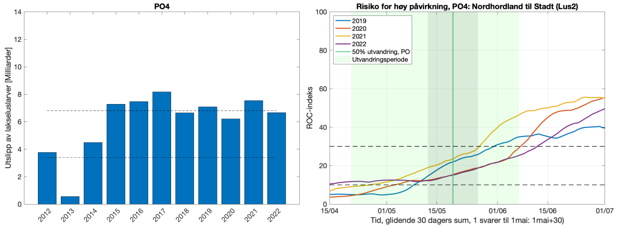
Figur 6.45. Venstre side viser utslipp av lakselus fra alle aktive oppdrettsanlegg i produksjonsområdet summert fra 4 uker før til 3 uker etter median smoltutvandring, der horisontale stiplete linjer indikerer grensene for høyt og lavt utslipp. Høyre side viser ROC indekser for fisk som står i fjorden fra dato på x-aksen og 30 dager frem i tid. Grafen skal leses sammen med ROC kartet (Figur 6.46) og verdiene i grafen viser andelen av arealet med forhøyet tetthet av smittsomme luselarver (jfr. Modellmetode 1: ROC). Heltrukken vertikal linje markerer tid for median utvandring, grønt areal utvandringsperioden for postsmolt av laks brukt i den virtuelle smoltmodellen. Horisontale stiplete linjer markerer 10 og 30% areal.
