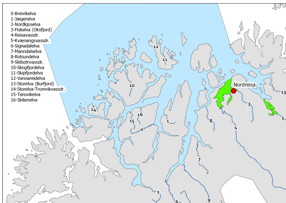
Figur 6.135. Stasjonene undersøkt minst tre av årene i perioden 2016-2022 i NALO programmet. Straumfjord og Øksfjord er slått sammen og kalt Nordreisa. Lakseelvene i området er vist som tall i kartet. Grønt areal indikerer nasjonale laksefjorder.
