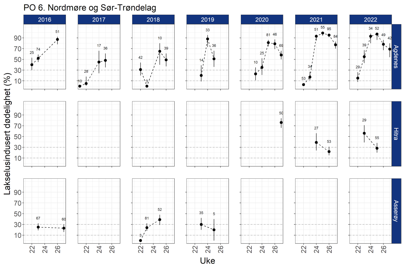
Figur 6.82. Estimert lakselusindusert dødelighet (%) med konfidensintervaller på alle stasjonene undersøkt. Beregningene inkluderer all fisk fanget. Antall sjørørret undersøkt hver uke er angitt i figuren.
