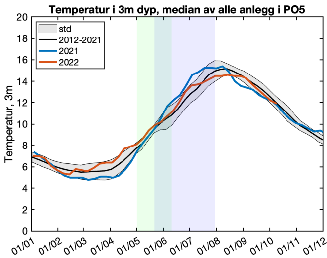
Figur 6.58. Median temperatur på 3 m dyp basert på rapporterte temperaturer på oppdrettsanlegg i produksjonsområdet. Svart linje viser snitt av årene 2012-2022 hvor standardavvik er markert med grått felt, samt temperaturen i 2021 (blå linje) og 2022 (rød linje). Grønt område viser antatt utvandningsperiode for laks, blått antatt beiteperiode i sjø for sjørørret som vandrer ut på tidspunktet for 50% utvandring av laksesmolt.
