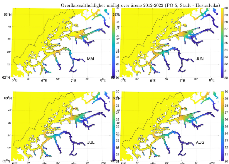
Figur 6.59. Utbredelse av saltholdighet i overflaten midlet for årene 2012-2022 i mai, juni, juli og august. Verdiene er beregnet vha. strømmodellen NorKyst800.
