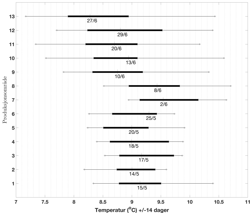
Figur 6.2. Temperatur under smoltutvandringen. Fordelingen av middeltemperatur (2012-2022) for arealet innenfor grunnlinjen i hvert produksjonsområde på ca. 0,5m dyp for tidspunkt rundt midtpunkt for smoltutvandringdatoen ( \pm 14 dager). Denne datoen er vist på hver linje under median temperatur. Tykk svart strek angir spennet mellom kvartilene (25% og 75%), mens tynn strek angir minimums- og maksimumsverdier. Vertikalaksen angir produksjonsområdene fra sør (1) til nord (13).
