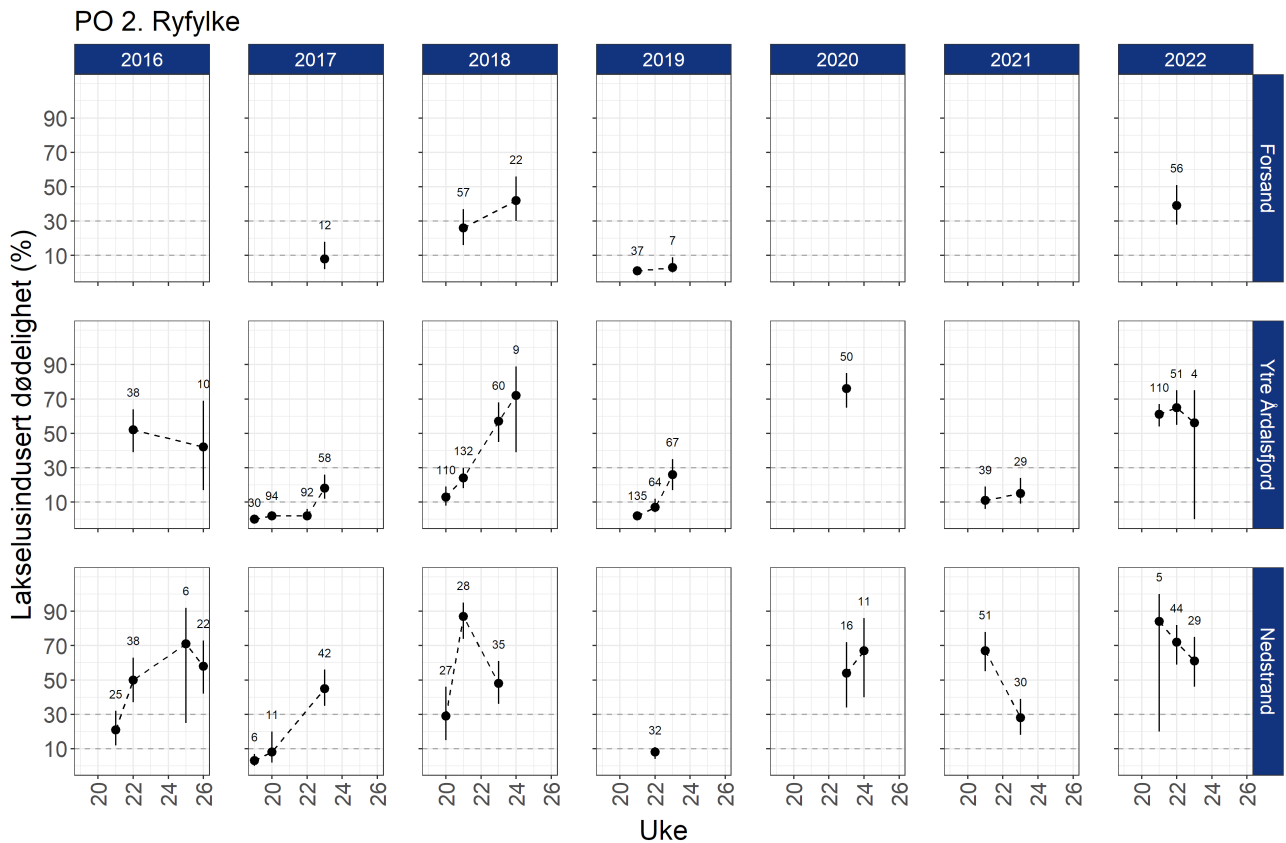
Figur 6.22. Estimert lakselusindusert dødelighet (%) med konfidensintervaller på alle stasjonene undersøkt. Beregningene inkluderer all fisk fanget og alle lusestadier. Antall sjøørret fanget hver uke er angitt i figuren.
