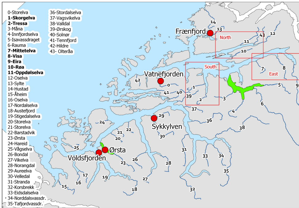
Figur 6.66. Stasjonene undersøkt minst tre av årene i perioden 2016-2022 i NALO programmet. Lakseelvene i området er vist som tall i kartet, utheverte elver er brukt til genetisk sporing av hjemelv for trålfanget laks fra området. De røde rektanglene omslutter elvene som renner ut i sørlige, østlige eller nordlige deler av Romsdalsfjorden. Grønt areal indikerer nasjonale laksefjorder.
