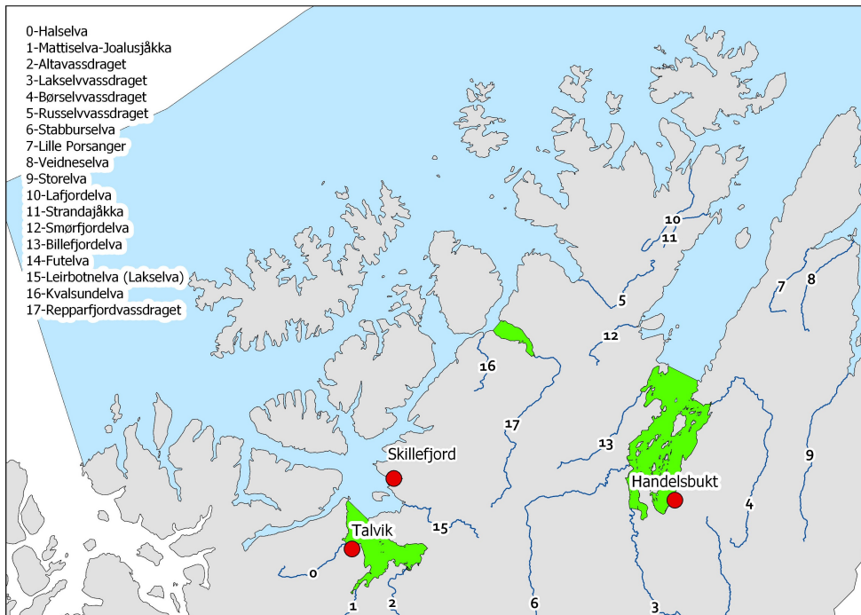
Figur 6.145. Stasjonene undersøkt minst tre av årene i perioden 2016-2022 i NALO programmet. Lakseelvene i området er vist som tall i kartet. Grønt areal indikerer nasjonale laksefjorder.
