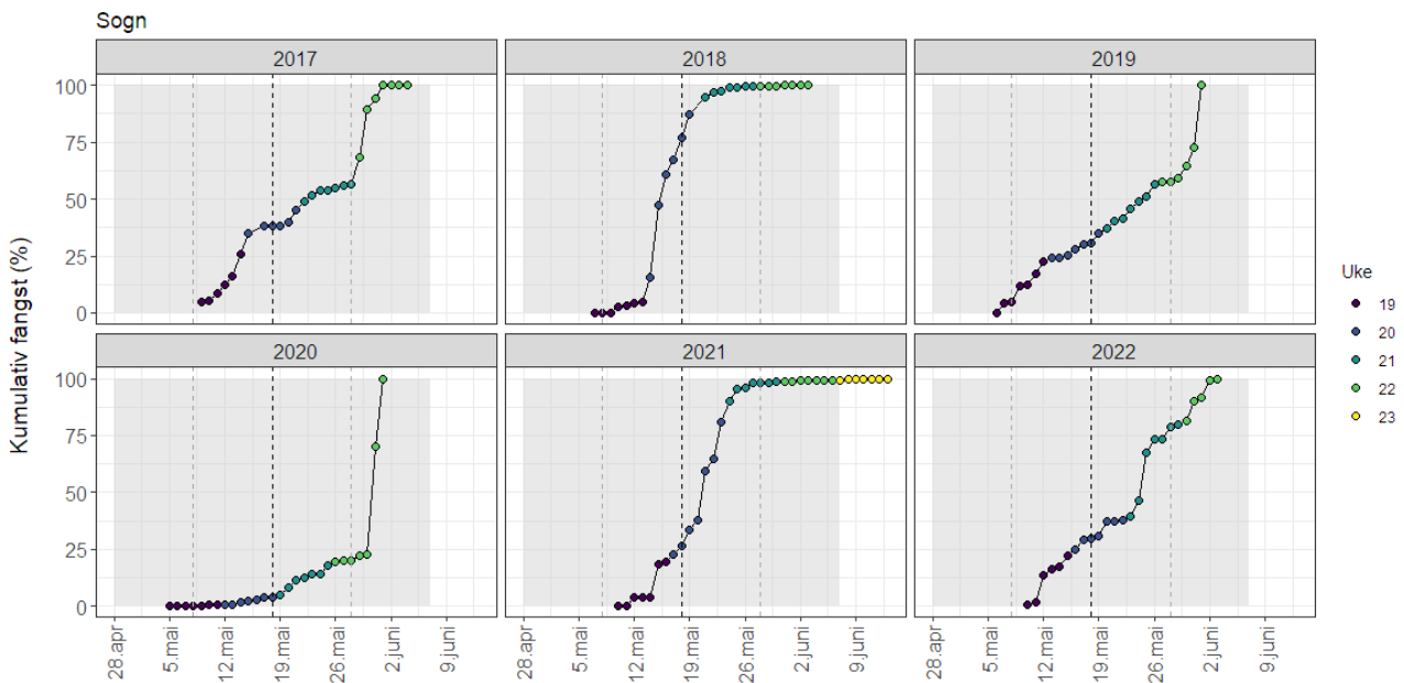
Figur 6.54. Kumulativ fangst av laksesmolt i trål i Sognefjorden 2017-2022 som % av totalfangst.
