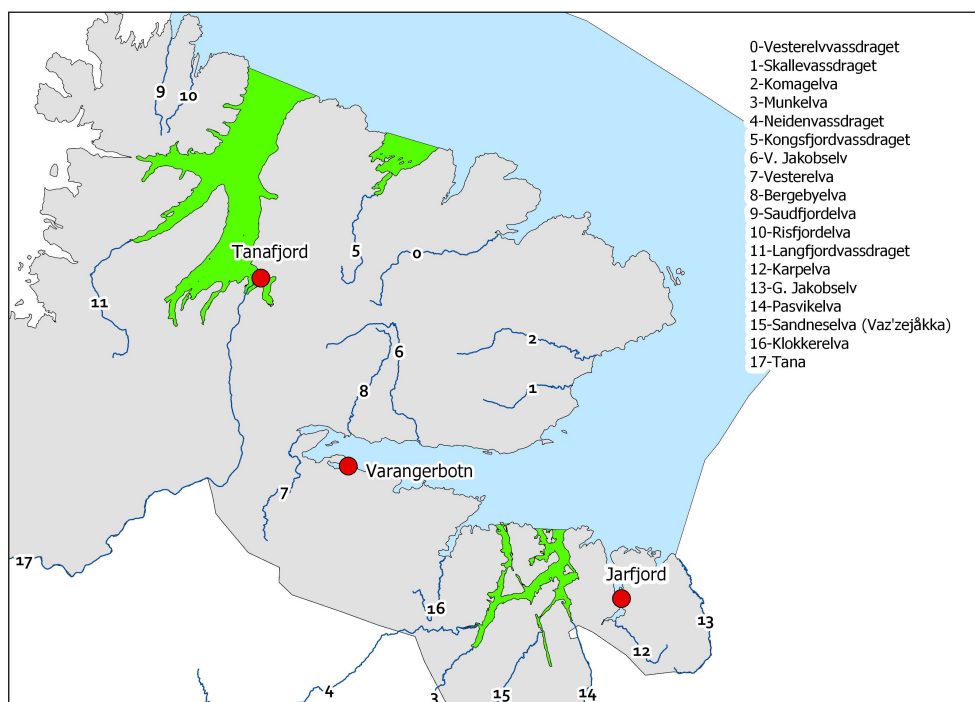
Figur 6.157. Stasjonene undersøkt minst tre av årene i perioden 2016-2022 i NALO programmet. Lakseelvene i området er vist som tall i kartet. Grønt areal indikerer nasjonale laksefjorder.
