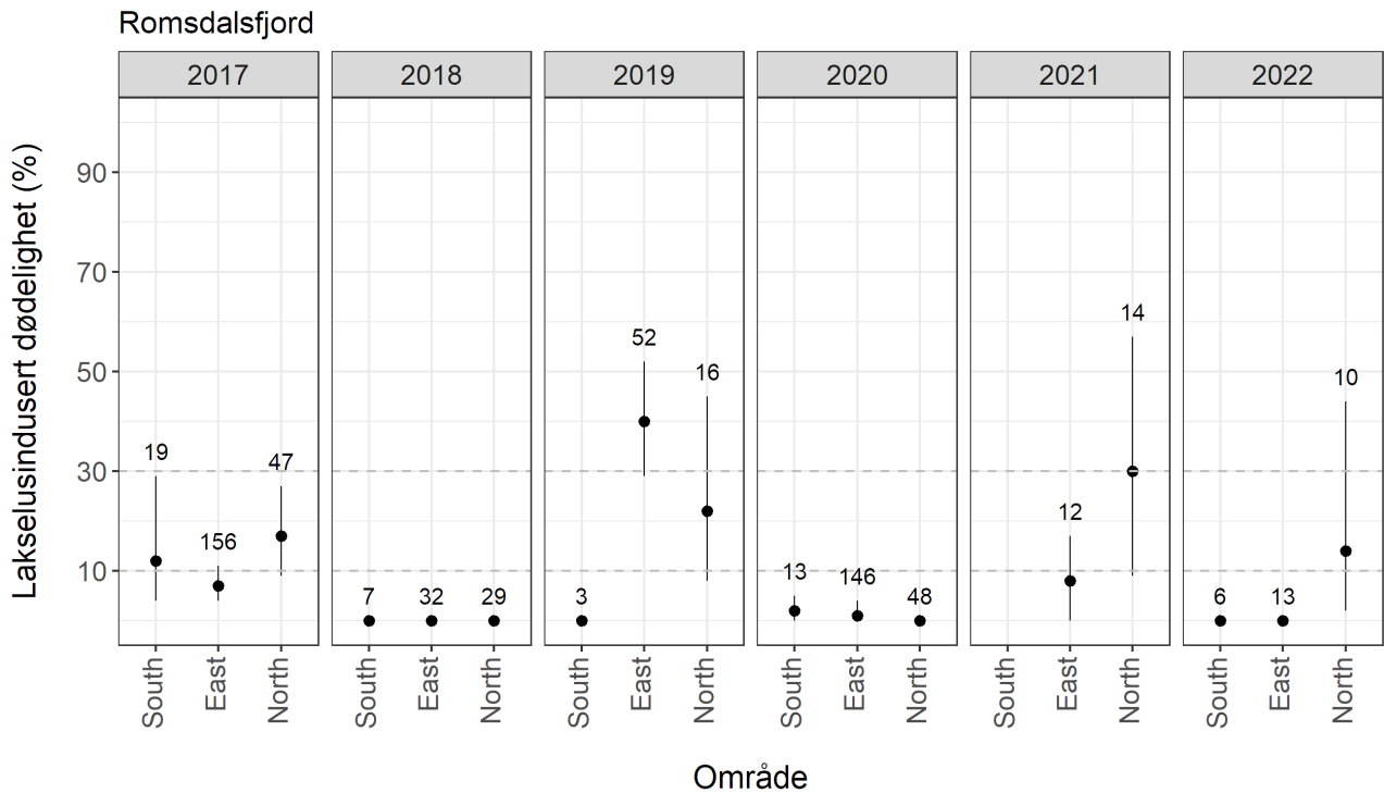
Figur 6.71. Estimert lakselusindusert dødelighet (%) med konfidensintervaller på trålfanget vill postsmolt av laks tilordnet hjemmelv. Elver som kan tilordnes er vist i Figur 6.66. Antall laks analysert er angitt i figuren.
