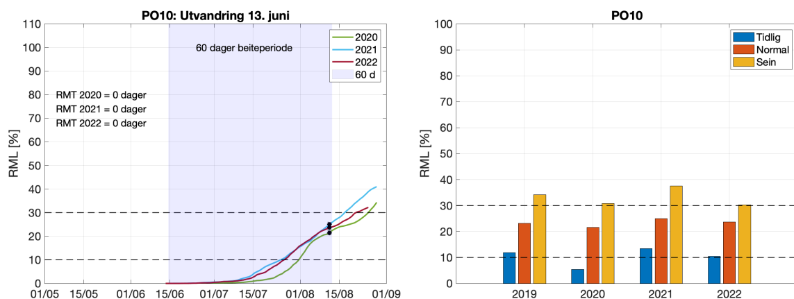
Figur 6.121. Venstre figur viser kumulativt redusert marint leveområde (RML) for fisk som utvandrer ved median dato for utvandring for alle elvene i produksjonsområdet og redusert marin beiteperiode (RMT) 2020-2022 (tekst i figuren). Skravert område indikerer antatt naturlig beiteperiode (60 dager). Høyre figur viser RML etter 60 dager for årene 2019-2022 ved median dato for utvandring (Normal), og ved 20 dager tidligere (Tidlig) eller 20 dager senere utvandring (Sein).
