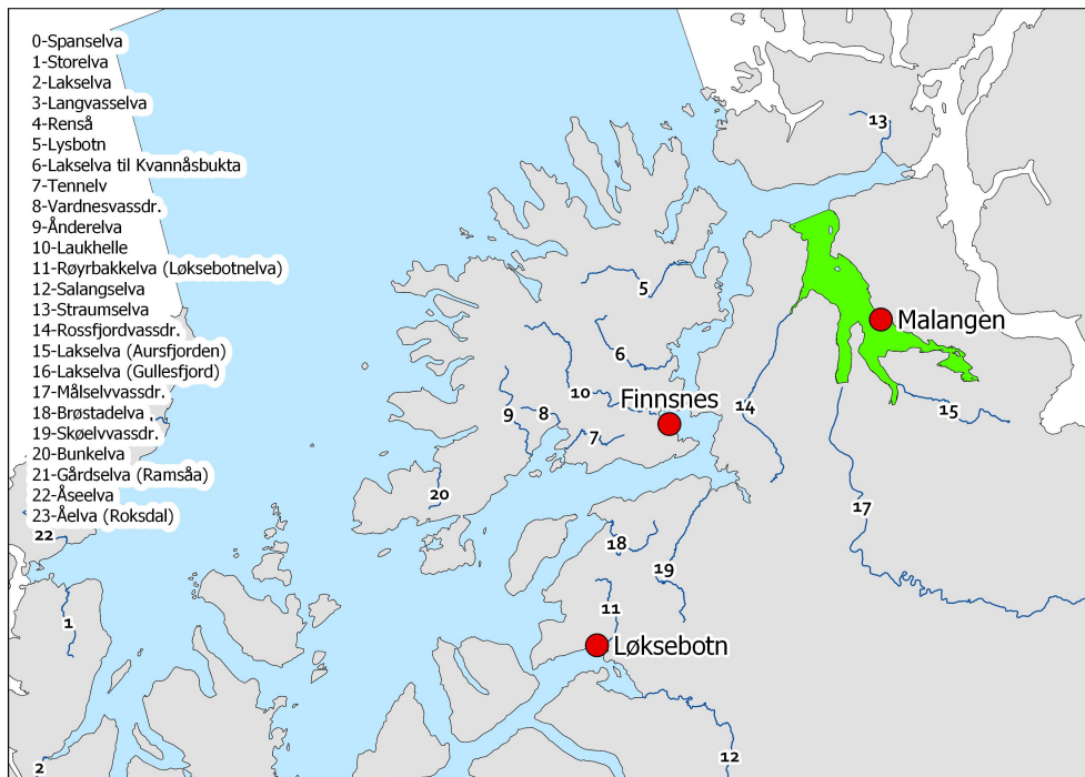
Figur 6.125. Stasjonene undersøkt minst tre av årene i perioden 2016-2022 i NALO programmet. Lakseelvene i området er vist som tall i kartet. Grønt areal indikerer nasjonale laksefjorder.
