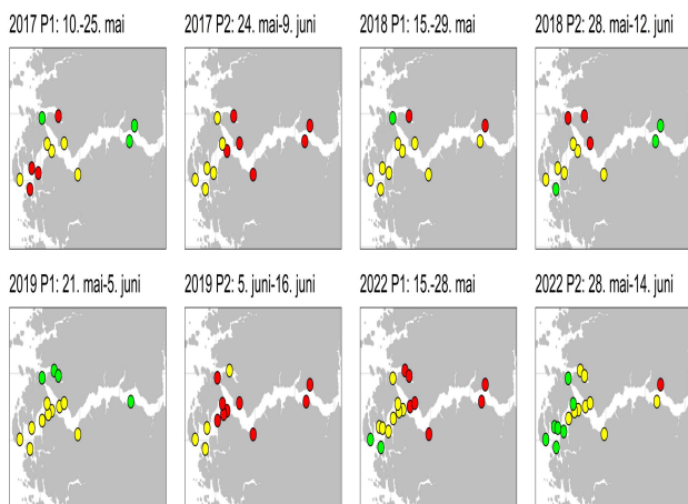
Figur 6.57. Snitt av antall lus/fisk normalisert til 14 dager for hver av smoltburene, fargene angir < 2 (grønne), 2-6 (gule), og > 6 lus/fisk (røde). Tidsperioden i figuren viser tiden burene stod ute.
