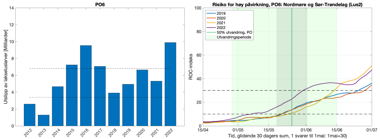
Figur 6.75. Venstre side viser utslipp av lakselus fra alle aktive oppdrettsanlegg i produksjonsområdet summert fra 4 uker før til 3 uker etter median smoltutvandring, der horisontale stiplete linjer indikerer grensene for høyt og lavt utslipp. Høyre side viser ROC indekser for fisk som står i fjorden fra dato på x-aksen og 30 dager frem i tid. Grafen skal leses sammen med ROC kartet (Figur 6.76) og verdiene i grafen viser andelen av arealet med forhøyet tetthet av smittsomme luselarver (jfr. Modellmetode 1: ROC). Heltrukken vertikal linje markerer tid for median utvandring, grønt areal utvandringsperioden for postsmolt av laks brukt i den virtuelle smoltmodellen. Horisontale stiplete linjer markerer 10 og 30% areal.
