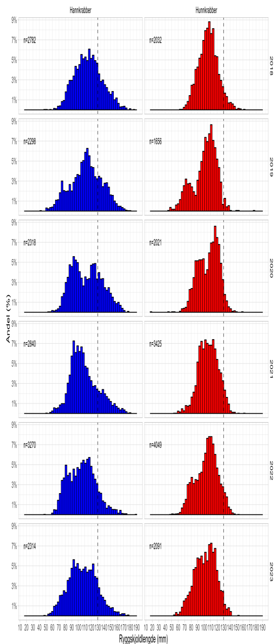
Figur 7. Relativ størrelsesfordeling hos hann- og hunnkongekrabber fra forskningstoktene 2018-2023. Stiplet vertikal linje angir minstemålet for fiske på 130 mm ryggskjoldlengde. N er den totale prøvemengden.
